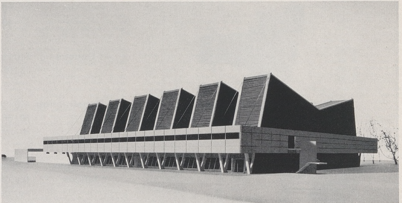
Hall des Sports à Landskrona - Vue générale de la maquette - Document : « L'Architecture d'Aujourd'hui », Paris
