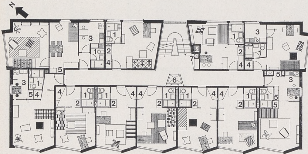
Plan type d'étage
